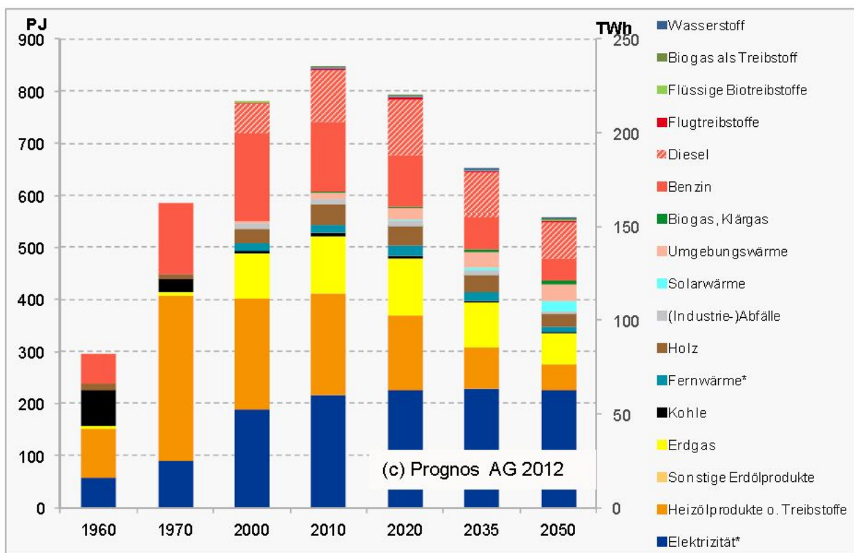
Grafik: Zusammensetzung des Endenergieverbrauchs (ohne Treibstoffverbrauch des internationalen Flugverkehrs) bis 2020, 2035, 2050 auf der Basis des Massnahmenpakets des Bundesrates (Quelle: Prognos)
